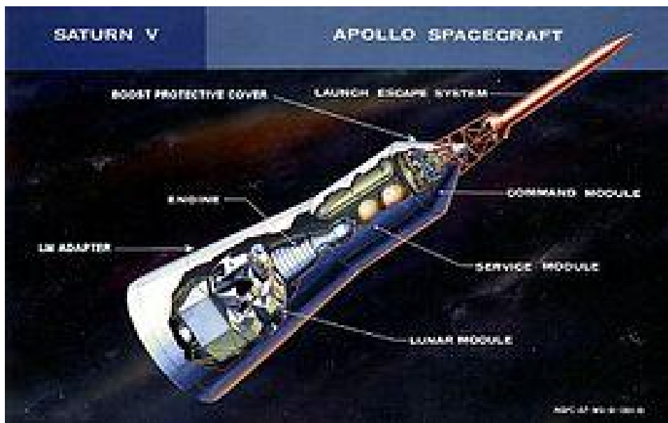
Command Module
